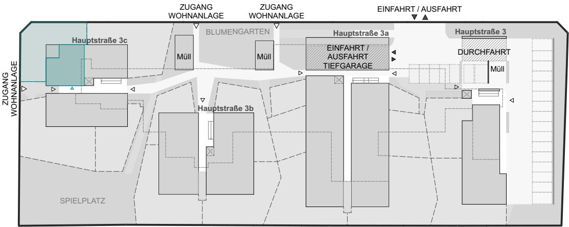
Übersichtsplan EG 0 1 2m
